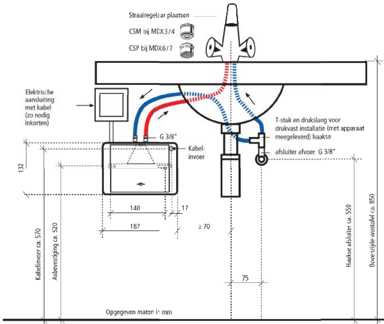
Montagevoorbeeld met druk vaste kraan
